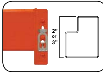
STEP LOAD BEAMS
